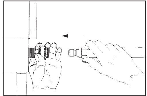
ILUSTRACIÓN #7 CONEXIÓN DE MANGUERA DE ALTA PRESIÓN
