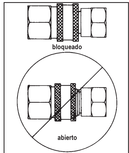
ILUSTRACIÓN #8 CONECTOR RÁPIDO
