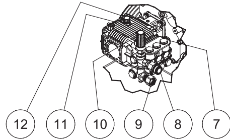
BOLT-ON UNLOADER
