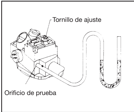
Ilustración #9 Ajuste Del Regulador De Gas
